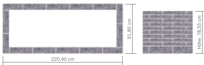
Seetaler Bruchsteinmauer BAUSATZ 2
